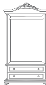
R769 ШКАФ 2-Х ДВЕРНЫЙ Д:1180 Г:640 В:2220
